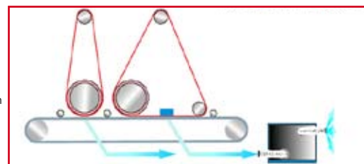
Zweipositions Schleifschuh mit Ab- und Zuflucht two-position pad with ascent and descent
